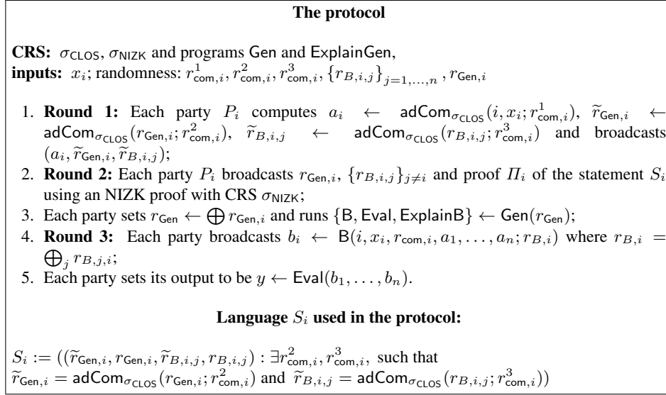
Fig. 6: Malicious MPC protocol.
