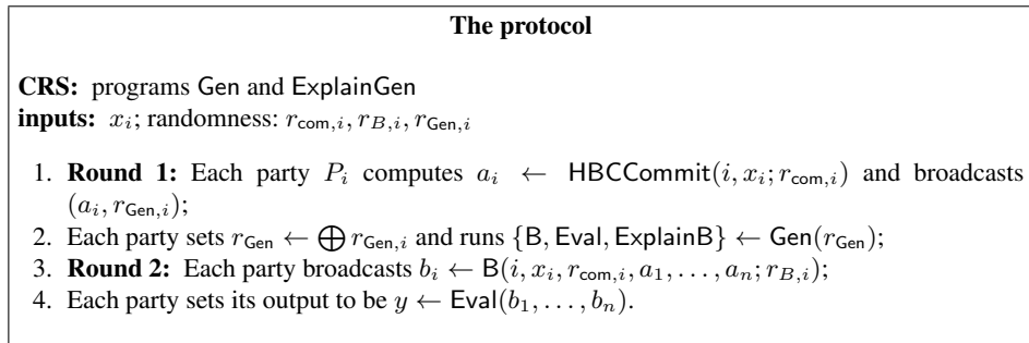
Fig. 2: MPC protocol.
