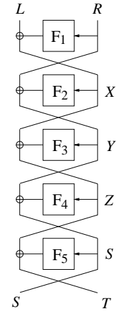
Fig. 4. 5-rounds Luby-Rackoff.
